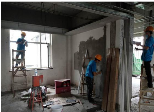
墙面抹灰
