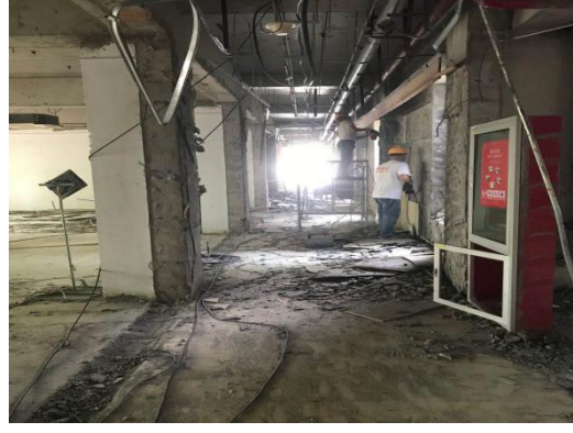
首层拆除
