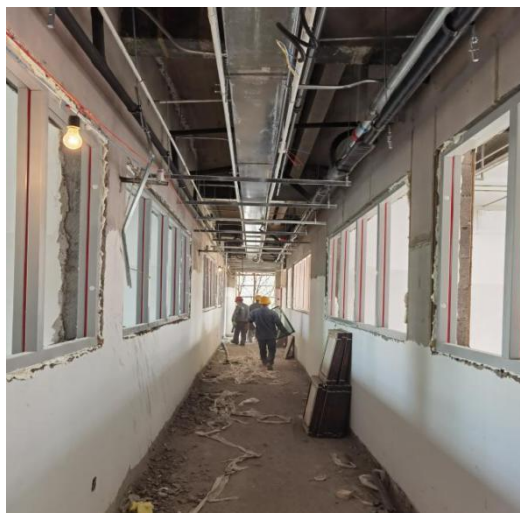
南段 3-4 层防火窗框安装
