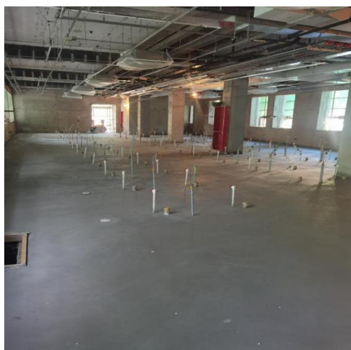
南段 1 层西侧地面施工
