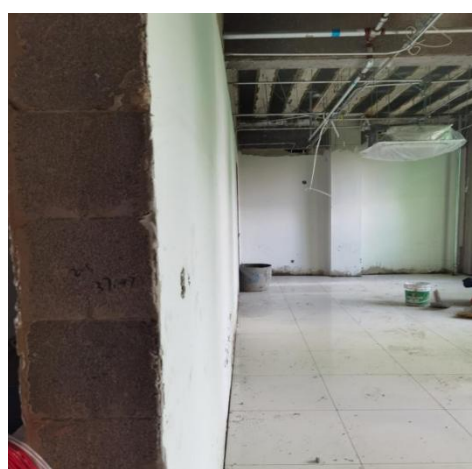
中段 2-4 层墙面施工
