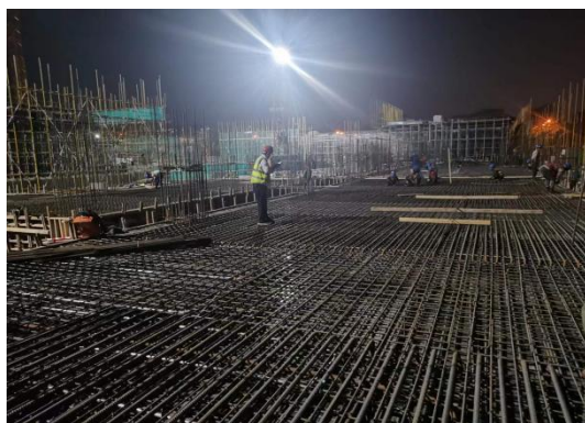
地下室顶板钢筋施工
