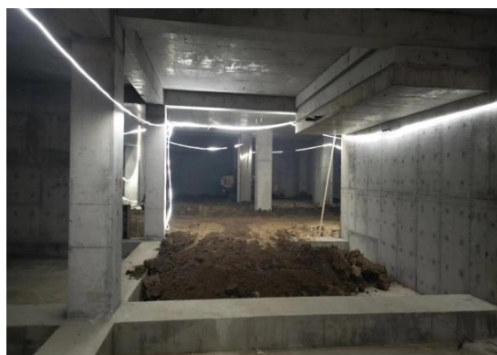
地下室内回填土施工
