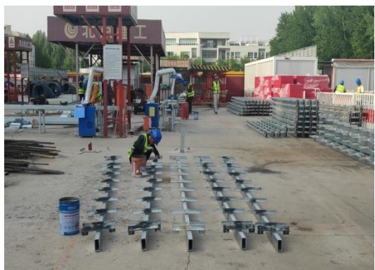
陶板幕墙龙骨加工
