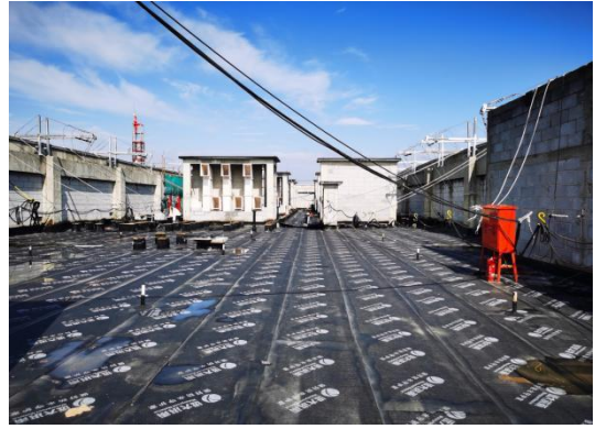
屋面防水施工
